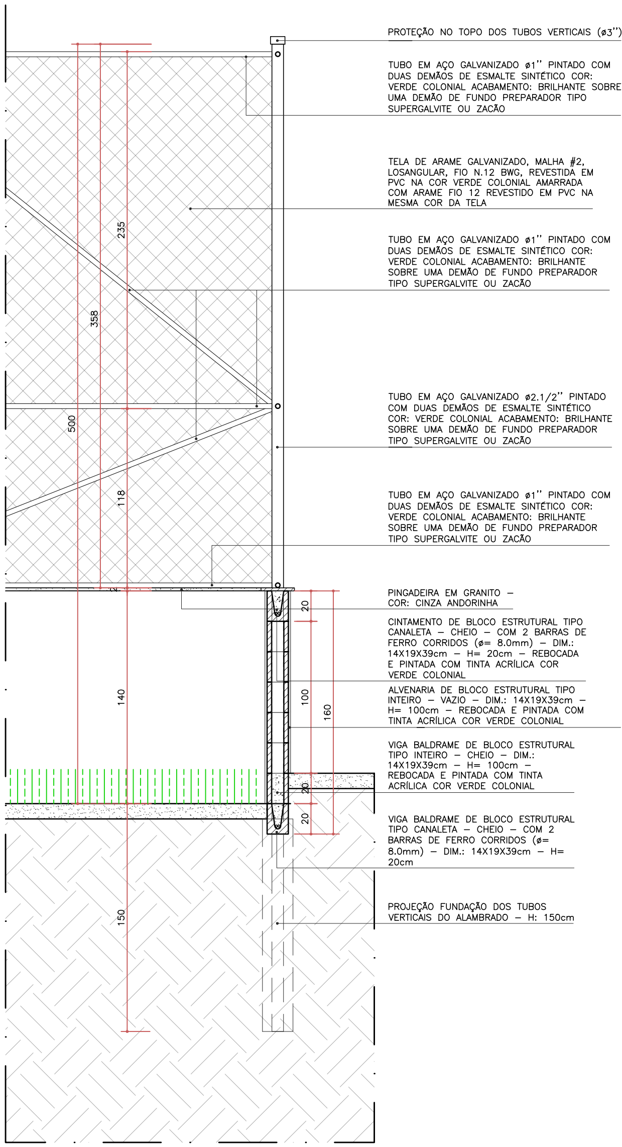
DETALHE - ALAMBRADO
