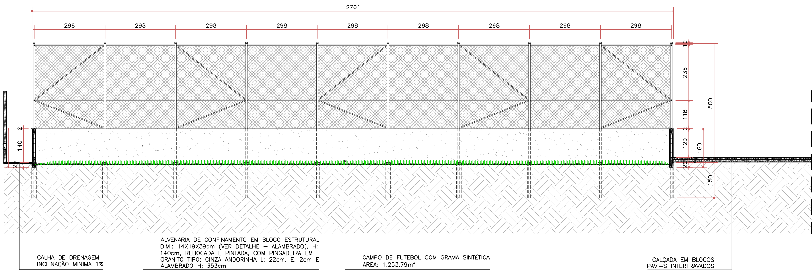
CORTE BB
