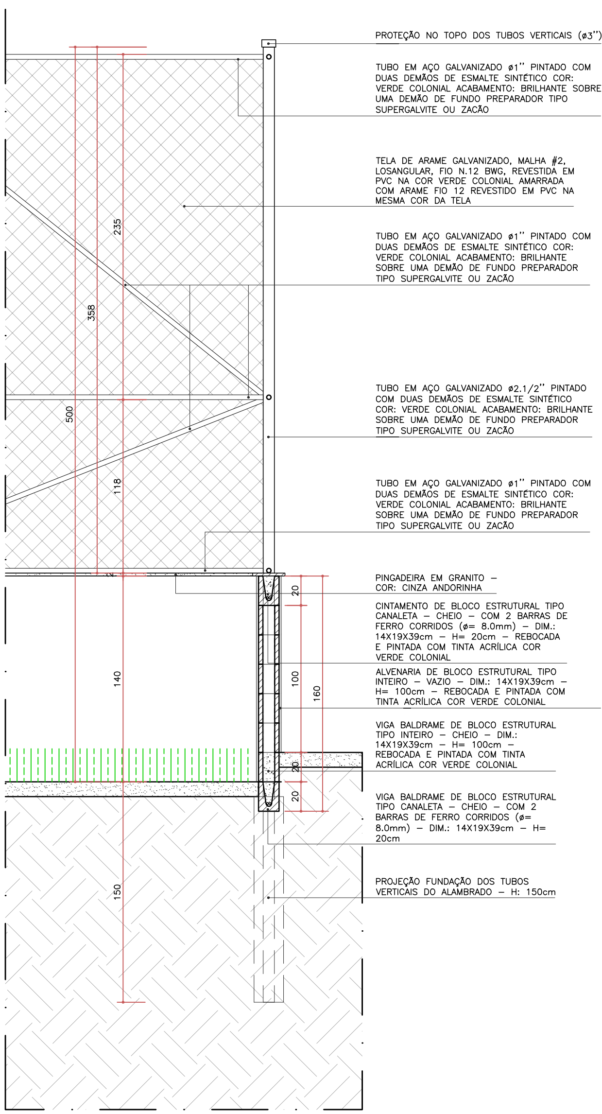
DETALHE - ALAMBRADO
