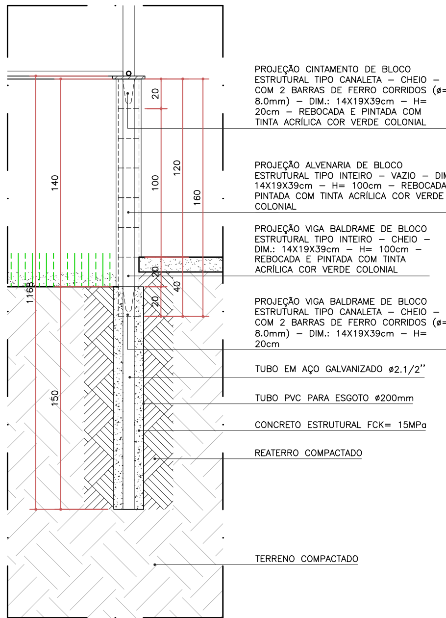
DETALHE - FUNDAÇÃO POSTE
