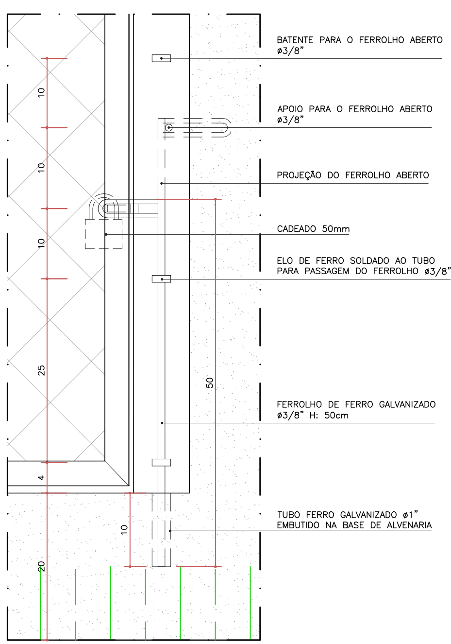
DETALHE - FERROLHO
