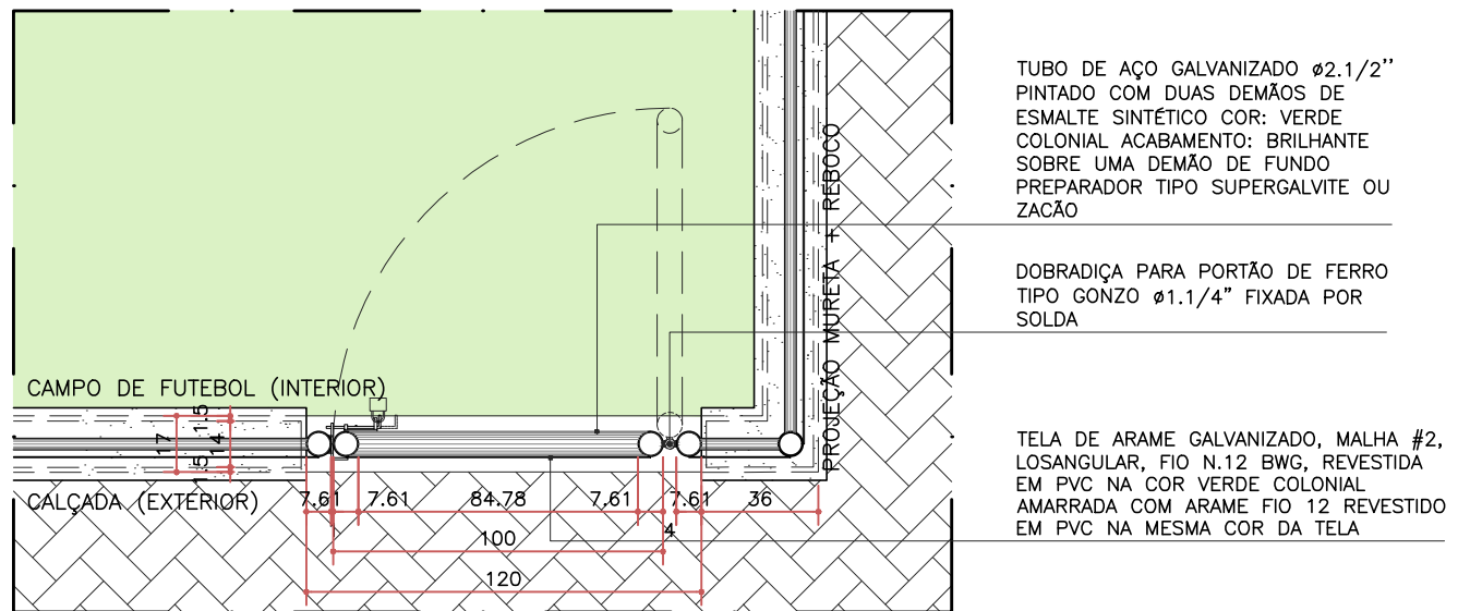
PLANTA BAIXA - PORTÃO
