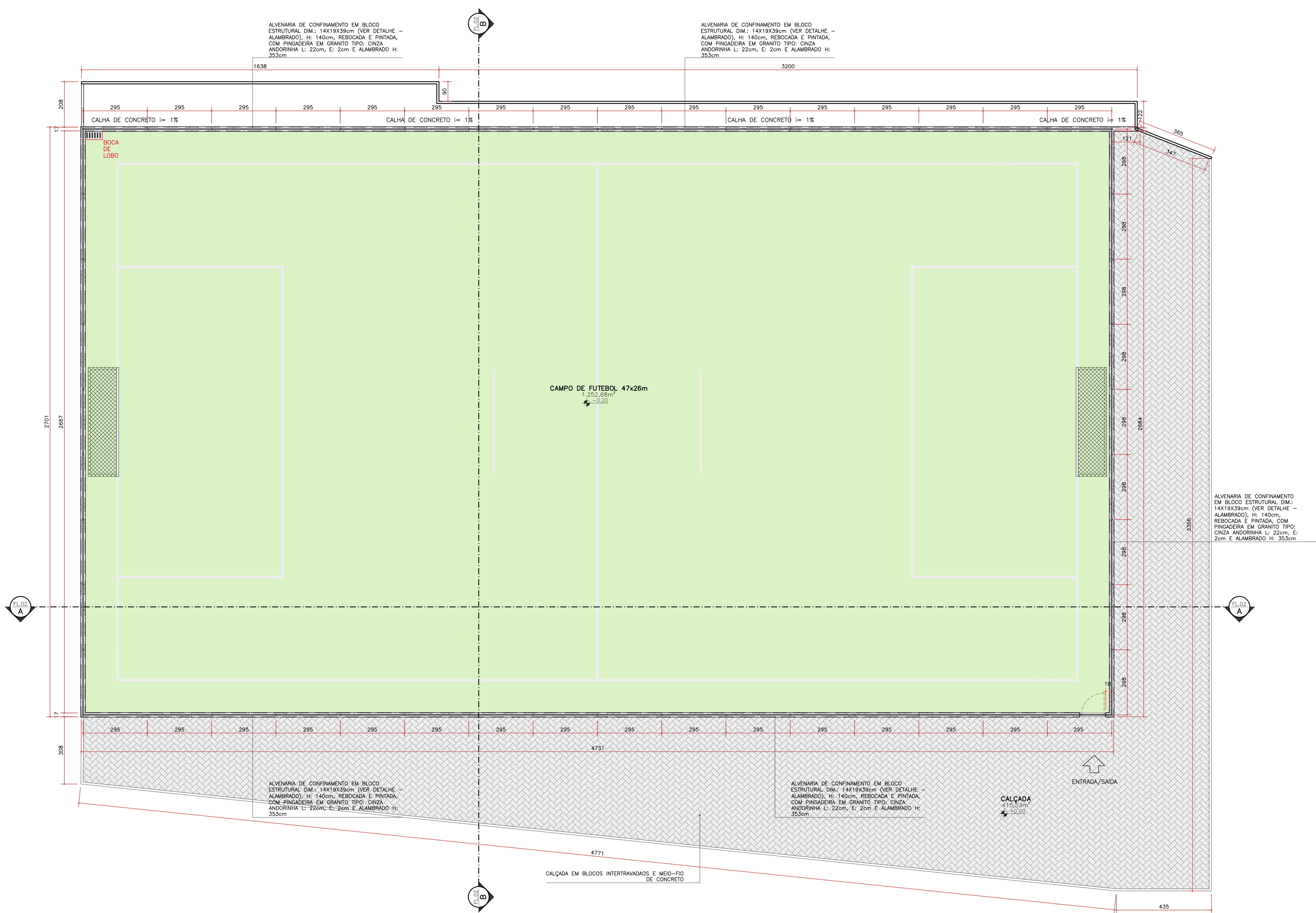
PLANTA BAIXA — CAMPO DE FUTEBOL (47x26m) ESG. 1:100
