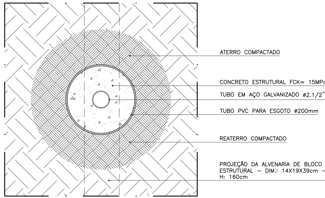
DETALHE - FUNDAÇÃO DO ALAMBRADO
