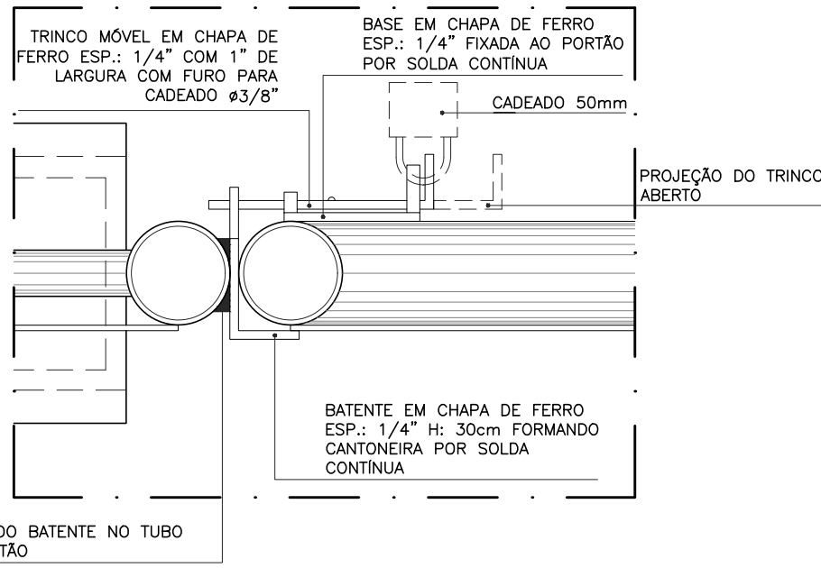
DETALHE - TRINCO MÓVEL
